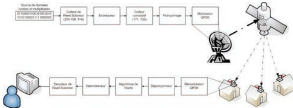
Figure 1 – Chaînes simplifiées d'émission et de réception satellite.
