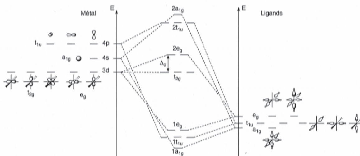
Figure 8 : Diagramme d'OM d'un complexe de symétrie octaédrique.
