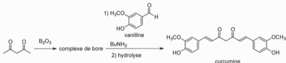
Figure 4 : Synthèse de la curcumine décrite par Pabon.
