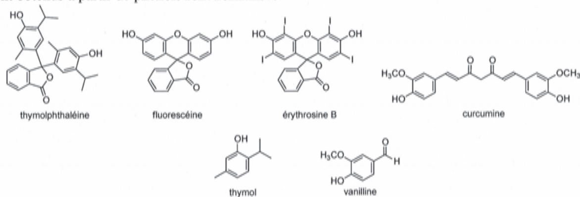
Figure 1 : Colorants et précurseurs.
