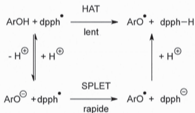
Figure 5 : Mécanisme de réaction de la curcumine avec le radical \text{dp}^{\bullet} .
